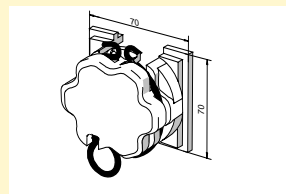
Крепление привода с пружинным кольцом
