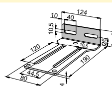
Кронштейн
