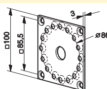
Фланцевое крепление привода
