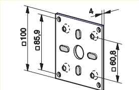
Фланцевое крепление привода с утолщениями
