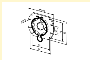
Крепление боковых крышек с пружинным кольцом
