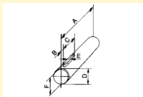
Приварной вал для устройства против срыва полотна TA O-RD/Z SOMFY
