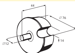
Ступица
