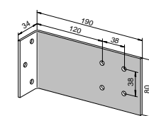
Кронштейн
