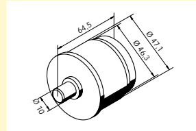
Ступица
