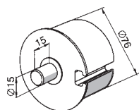
Ступица
