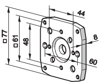
Универсальное крепление
