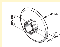
LT 50 Промежуточная пластина
