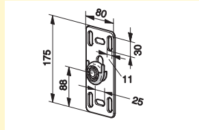
Фланцевая опора ступицы
