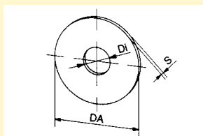
Круглая приварная заготовка для устройства против срыва полотна SOMFY
