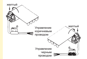
Кабель HiPro с наружным ограничительным выключателем
