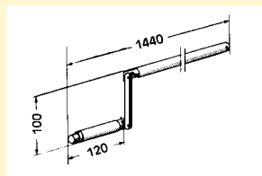
Шарнирный кривошип, несъемный
