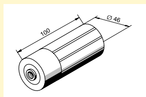
Регулируемая ступица без крепления
