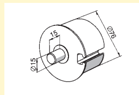
Ступица
