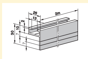
Шина С 112/А2 с вертикальной планкой
