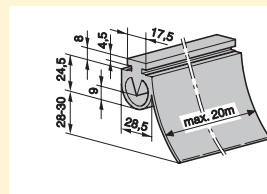
Стандартный контактный сдвоенный профиль с уплотнительной фаской
