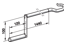
Шарнирный кривошип съёмный
