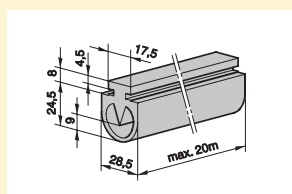
Стандартный контактный сдвоенный профиль
